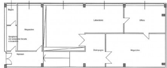
Piano seminterrato zona B - mq.220 scala 1:100
