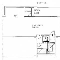
PIANO S2 h.2,40
