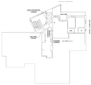
PIANO SETTIMO (H=2.70)
