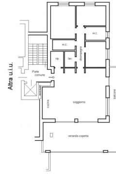
Piano Primo H = mt. 2,70
