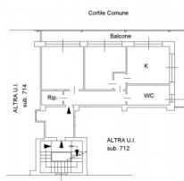
PIANTA PIANO PRIMO h: 295 cm
